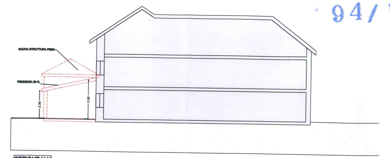
SEZIONE X-X
